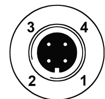
Femelle M12
