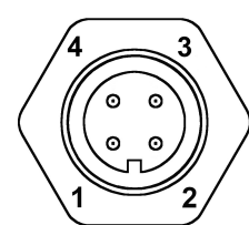
Mâle M12
